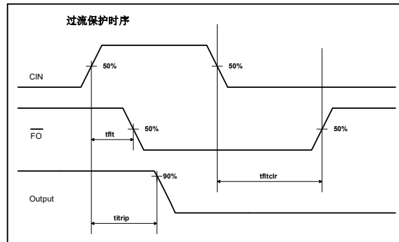
图 11 短路电流保护时序图 (只适合于低侧)
