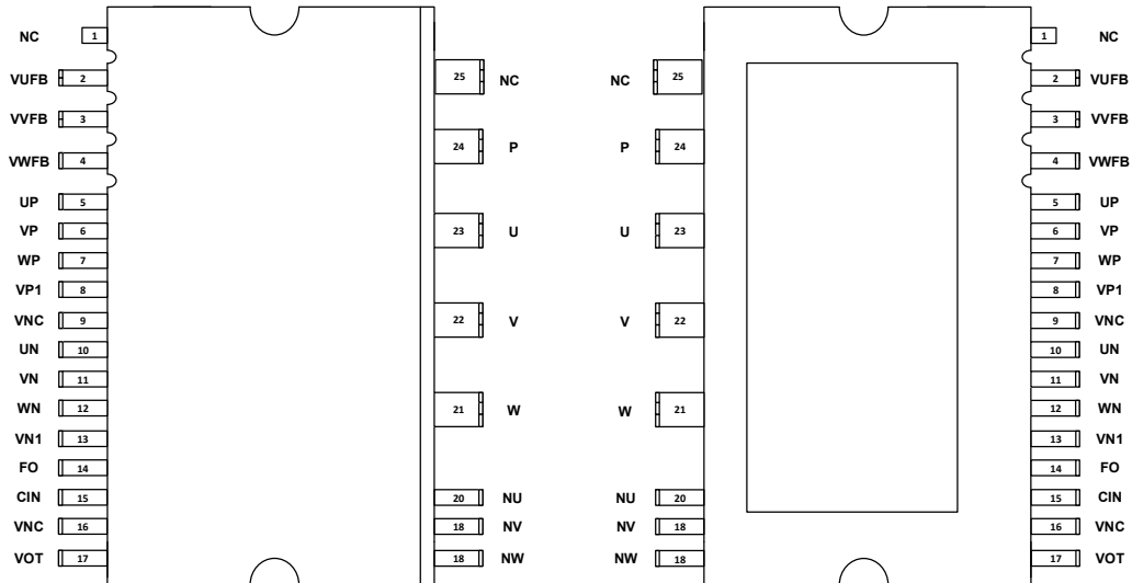
图 2 模块管脚定义
