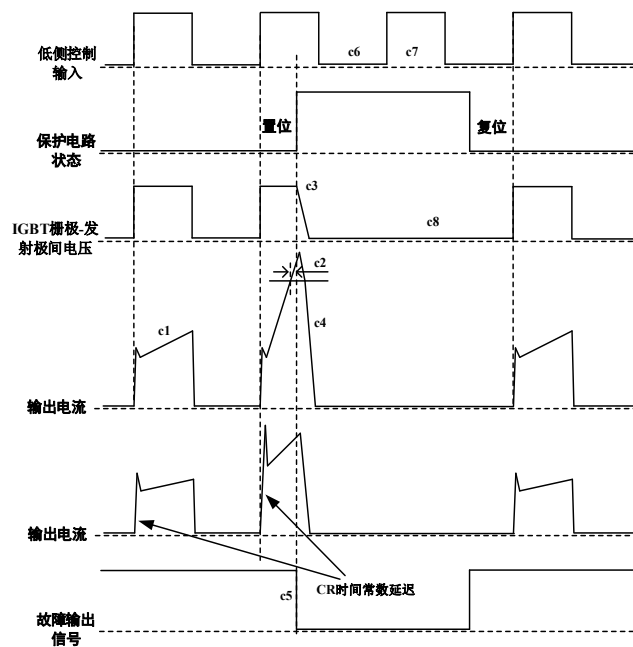
图 10 短路电流保护时序图(只适合于低侧)
